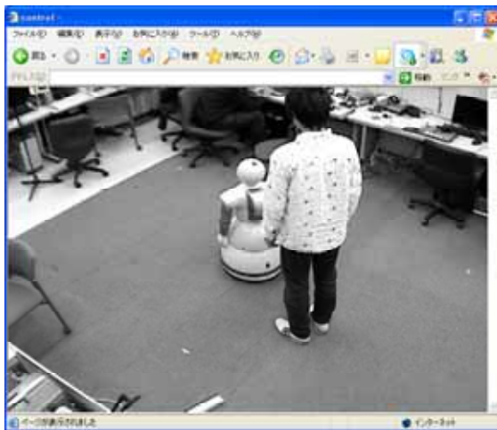
図5. 三人称視点
