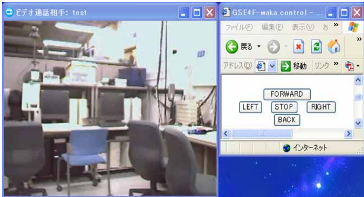
図4. 一人称視点
